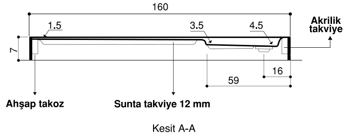
Monoblok Duş Teknesi
