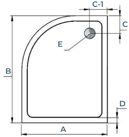
Sağ Gider / Right Drain
