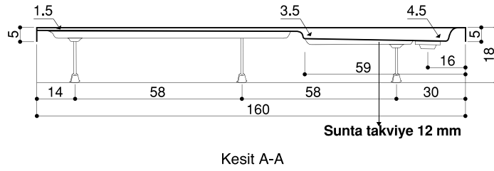
Ayaklı Duş Teknesi
