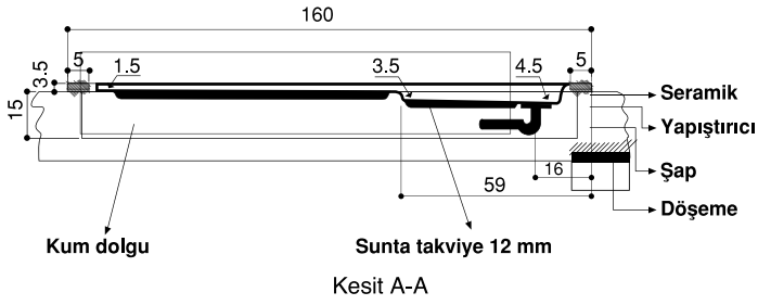
Flat Duş Teknesi
