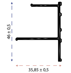
Agave Kanatlı Duvar Profili
