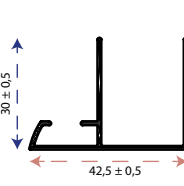
Agron - Amata Kanatlı Duvar Dikmesi
