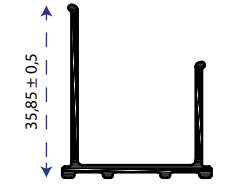
Agave-Agron-Amata Kapı Karşılık Duvar Profili
