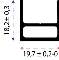
Altes Suluk Profili
