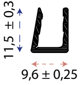
Akabe 571 U Çita 6 Mm
