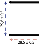
Aktor Kapı Karşılık Duvar Profili
