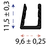
Akabe 571 - Aktor 6 Mm İçin U Profil
