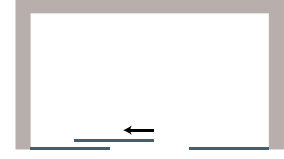
2 Sabit - 1 Kayar
