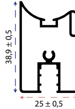
Aktor Menteşe Ayar Profili
