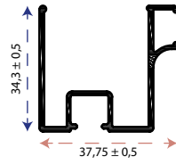
Agave Ayar Profili
