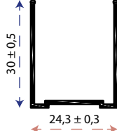
Agron - Amata Duvar Dikmesi
