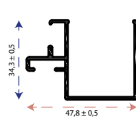
Agave-Agron-Amata Kapı Karşılık Profili
