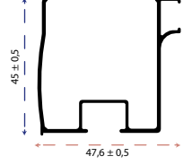
Limos 940 Ayar Profili
