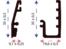
Çeneli Profil Ön - Arka Parça
