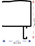
Arne Mıknatıslı Ayar Profili
