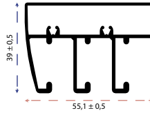
Alope 910 Üst Ray
